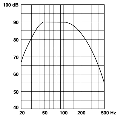
Diagram van de frequentie karakteristieken*
