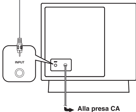
Pannello posteriore del subwoofer (Modelli per il Regno Unito e l'Europa)
