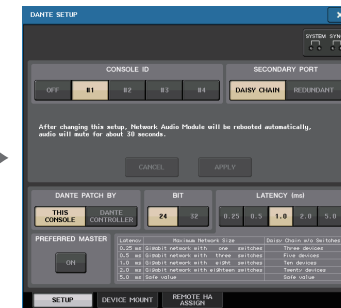
Janela DANTE SETUP
